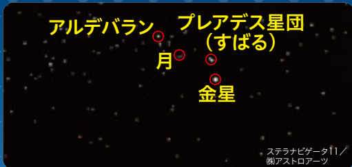
3月29日午後8時ごろの西の空
