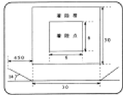
(ウ-2) 大型機(V-107及びUH-60J)の場合《応急》
