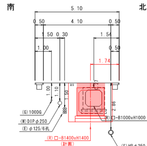
標準断面図
