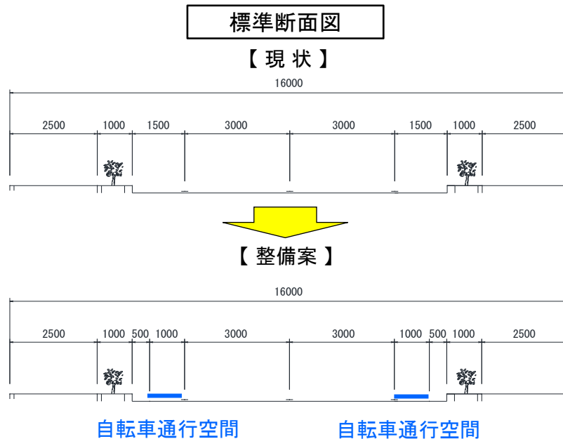
自転車通行空間の整備イメージ(矢羽根の設置)
