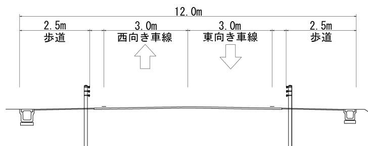
計画断面図
