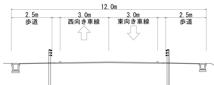
計画断面図
