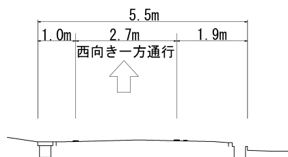
現況断面図
