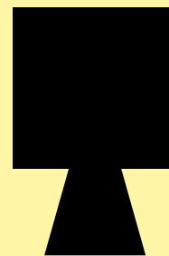
前方後方墳
