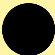
円墳
