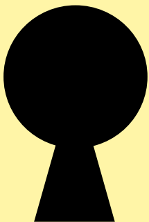
前方後円墳
