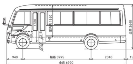
導入車両ロング（案）の図面
