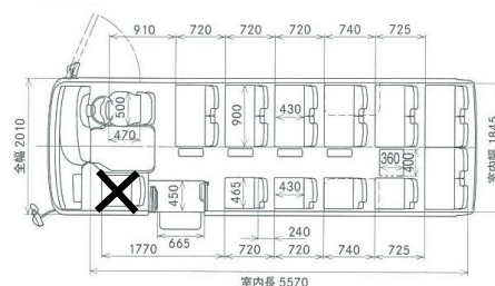
導入車両ショート（案）の図面
