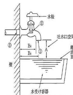
吐水口空間とは
