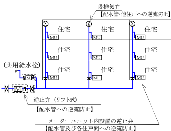
3階建て 集合住宅（各戸 貸与メーター）
