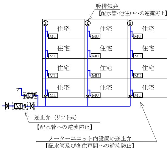
4階建て 集合住宅（各戸 貸与メーター）
