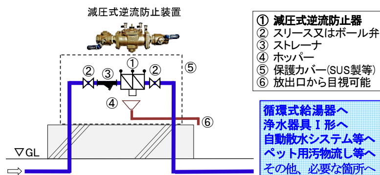
1 階地上設置の減圧式逆流防止器及び吸排気弁周りの配管要領図
