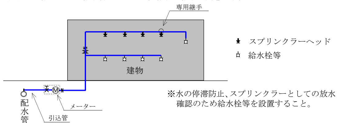
特定施設水道連結型スプリンクラー設備概要図
