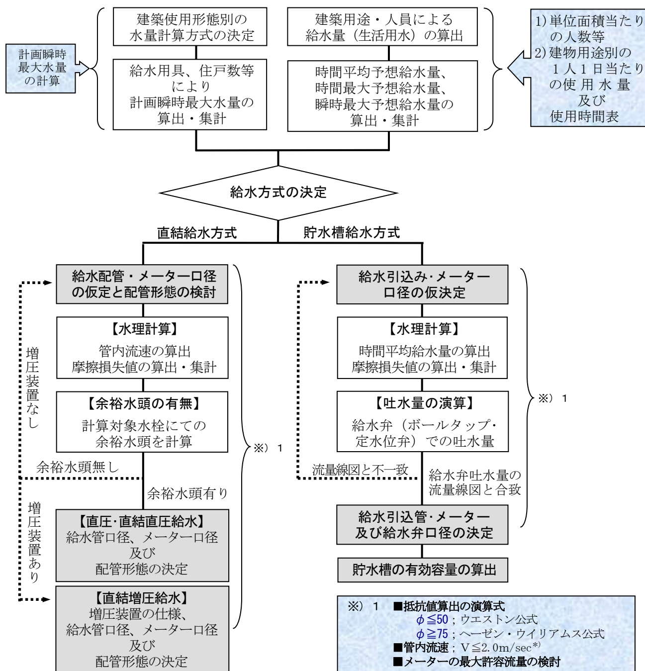
給水方式別の設計フロー
