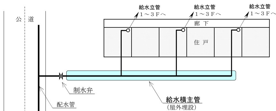
給水横主管と給水立管の概略図
