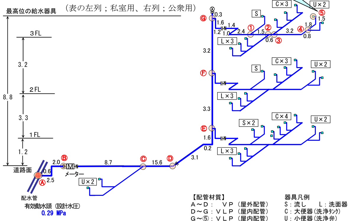
給水管の区間流量
