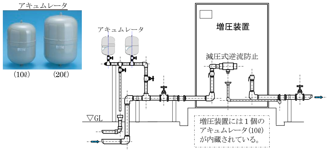
増圧装置一次側におけるアキュムレータ増設概要図
