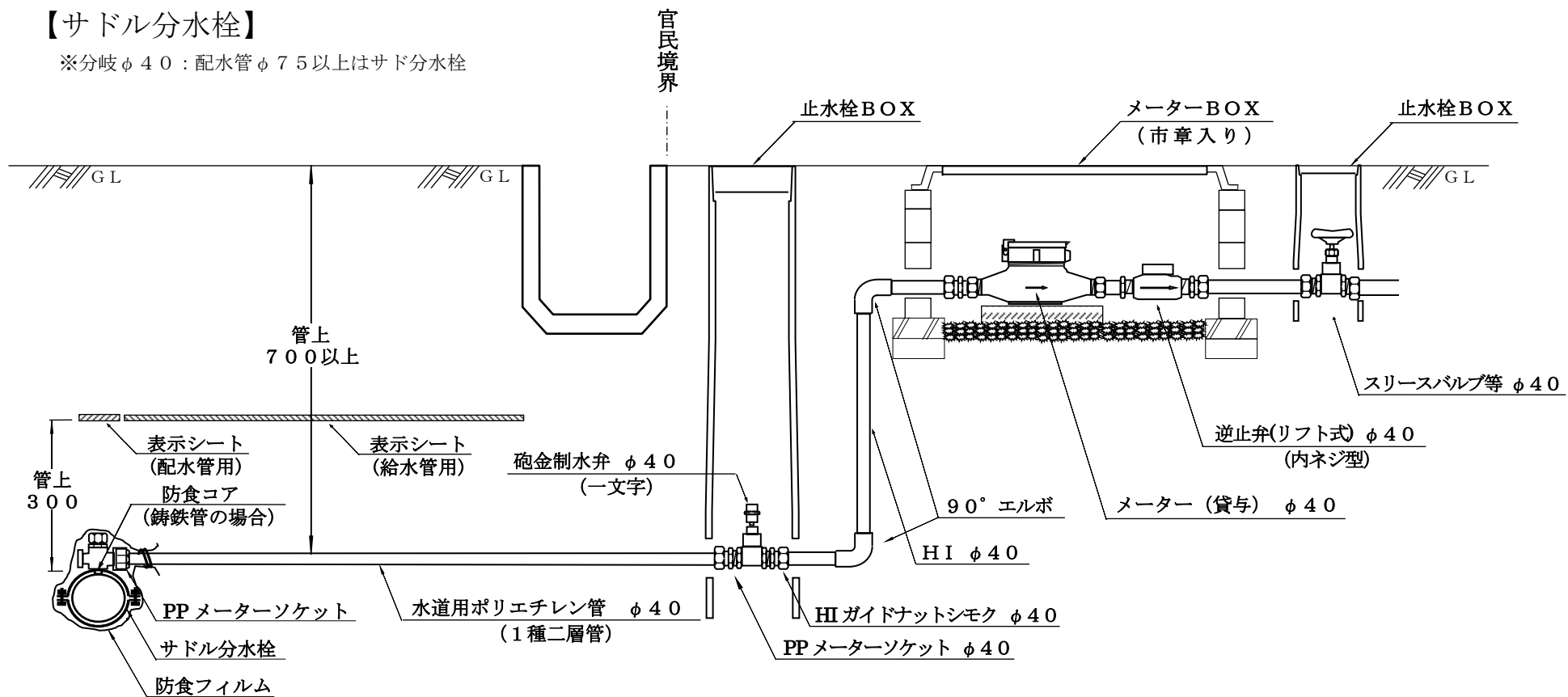
メーター口径 40 mm 給水管取出し及びメーター設置標準図
