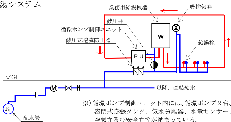
循環式給湯システムの概要図
