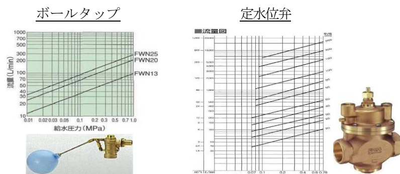
図3-1 流量線図
