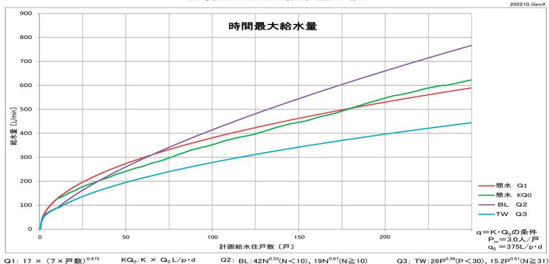
図 3－14 計算方式別給水量グラフ
