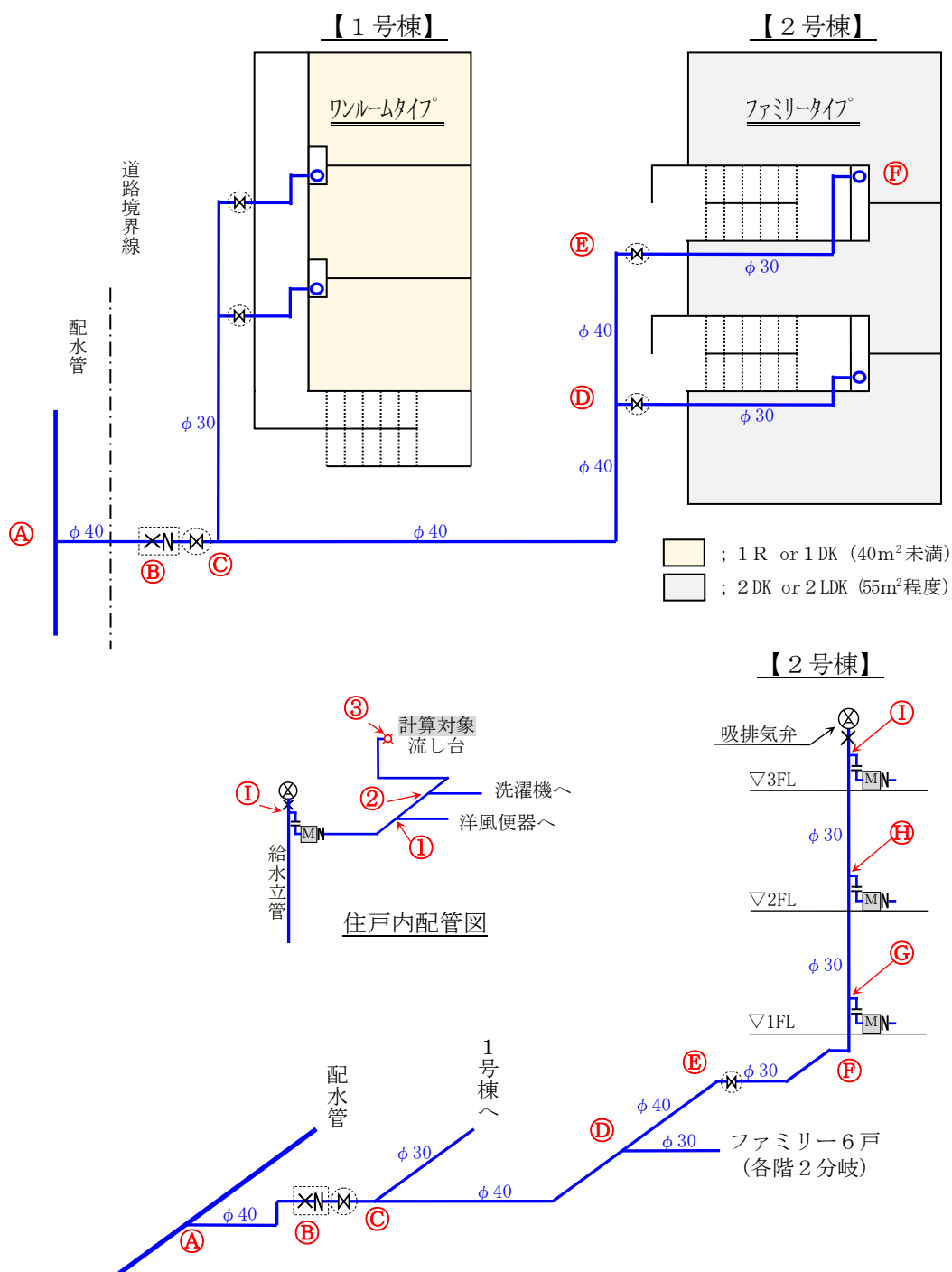
図6-3 3階建て集合住宅の平面・系統図
