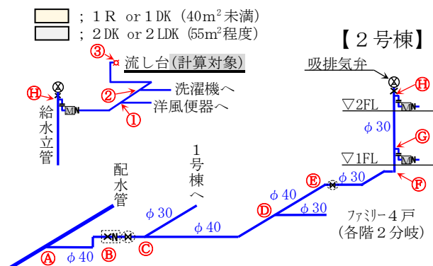
図3-7 系統図
