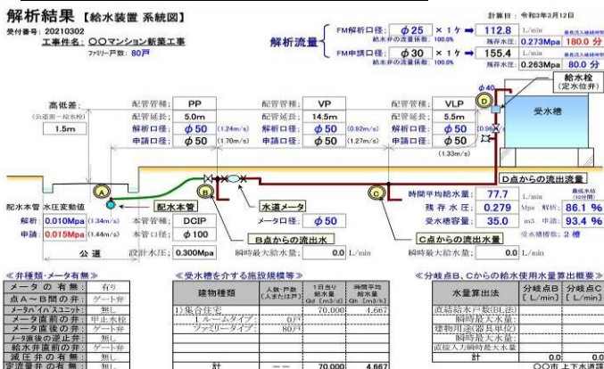
図6-17 設計水圧 0.300MPa(その2)
