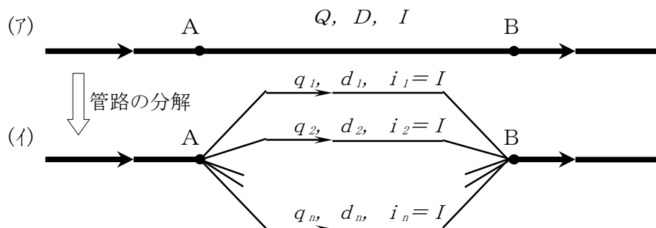
図 3 - 1 2 管路の平行閉管路への分解図 ( (ア) \Rightarrow (イ) )
