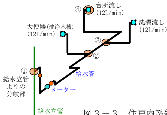
図3-3 住戸内系統図
