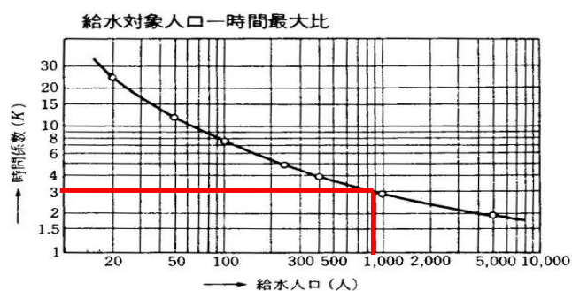
図3-13 計画時間最大配水量を求める為の時間係数：K
