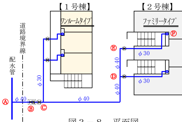
図3-8 平面図
