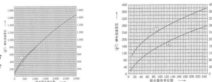
図3-10 器具給水負荷単位による流量線図
