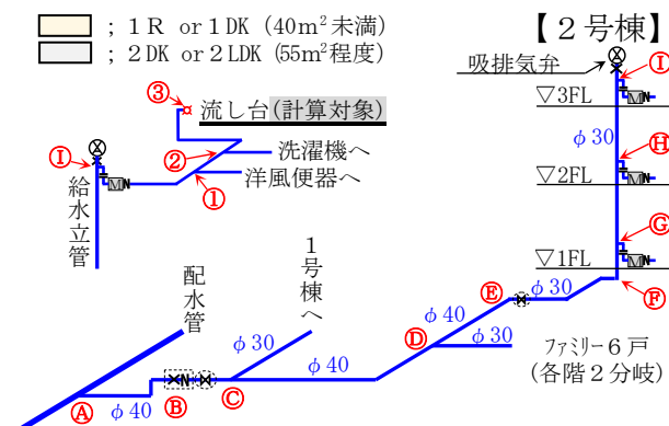
図3-9 系統図
