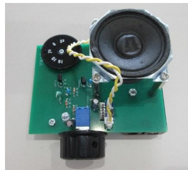
AM ラジオ
