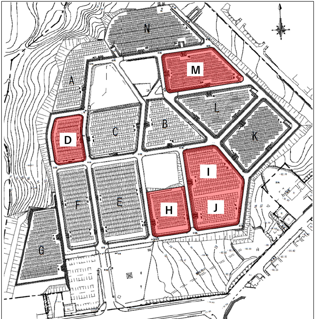
旭平和墓園区画内通路舗装工事 施工位置図
