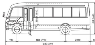
ロングボディ車両（案）の図面
