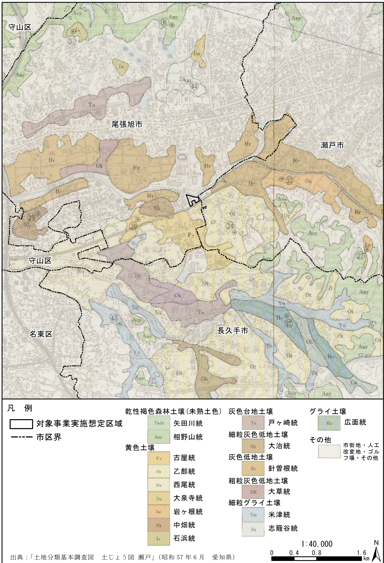
図 3.1.16 土壌図
