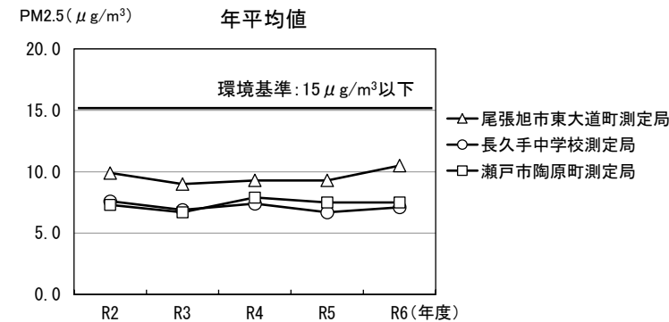
図 3.1.10 微小粒子状物質（年平均値）の経年変化
