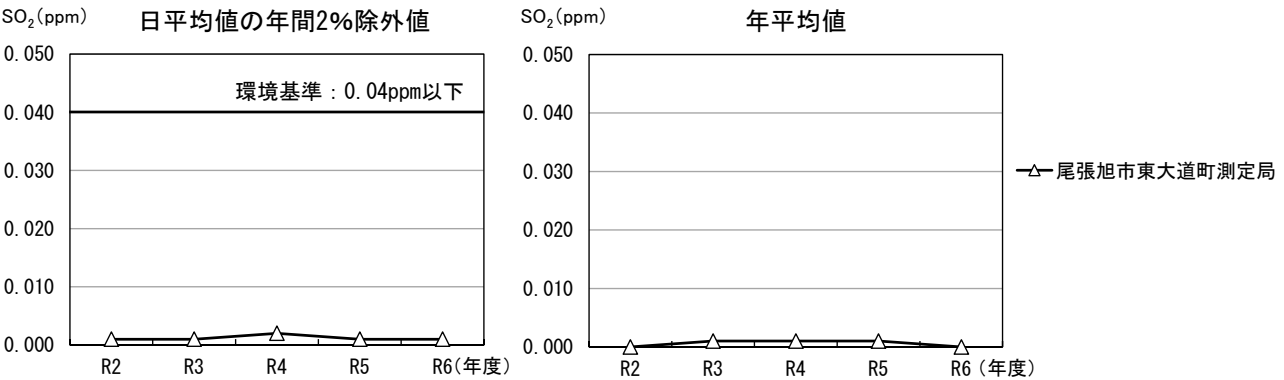
図 3.1.6 二酸化硫黄の経年変化
