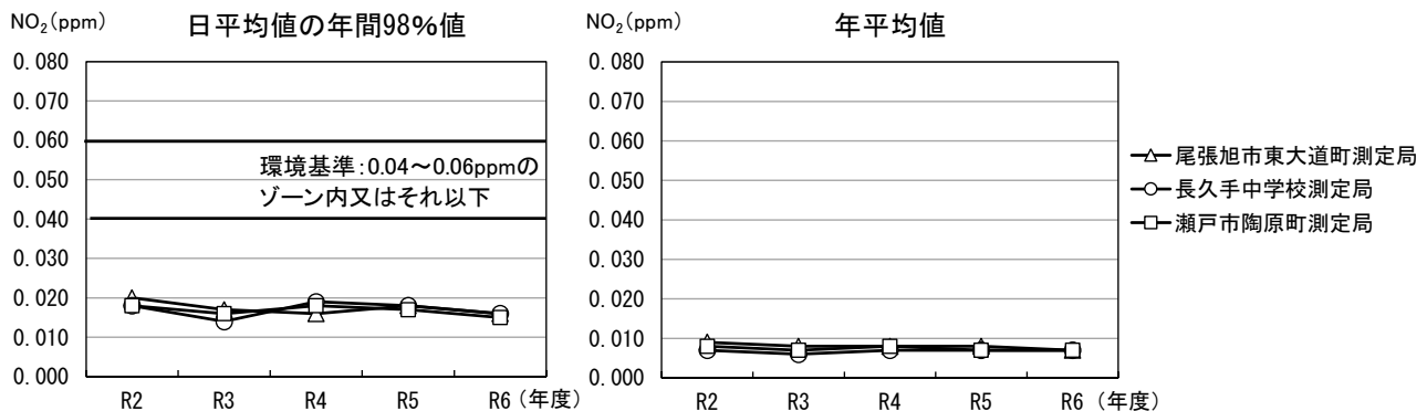
図 3.1.7 二酸化窒素の経年変化
