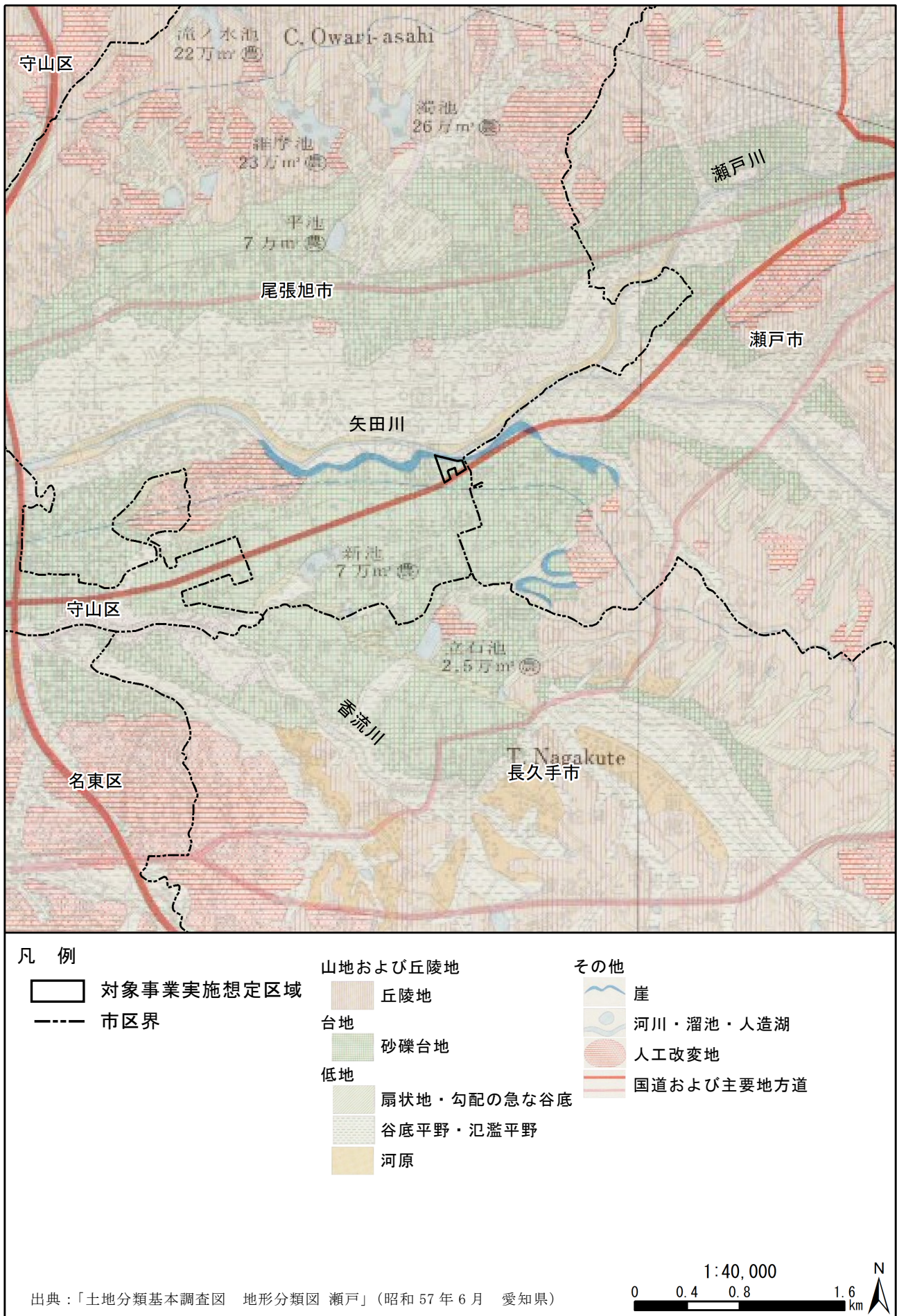
図 3.1.13 地形分類図
