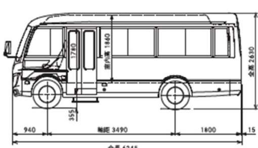
ショートボディ車両（案）の図面
