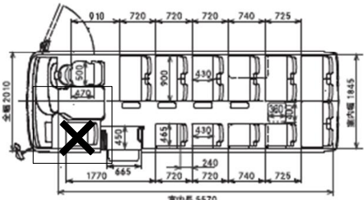
ショートボディ車両（案）の図面
