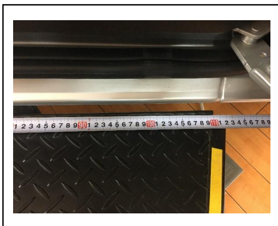
電動格納ステップの幅 (112 cm)
