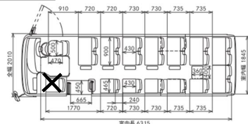
導入車両ロング（案）の図面
