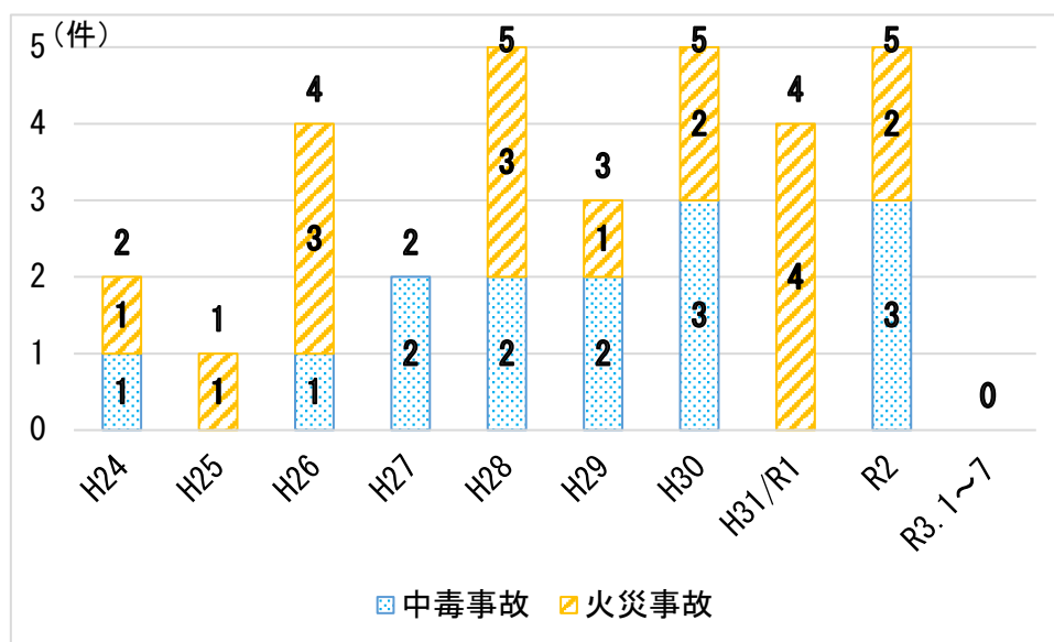
図4 発生年別携帯発電機事故件数
